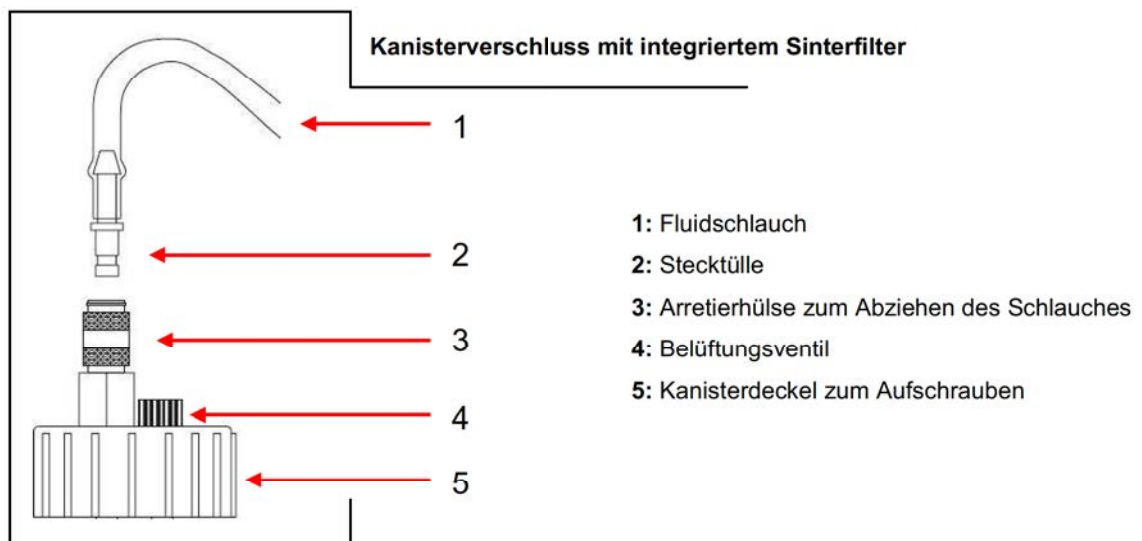
Abb. 4: Kanisterverschluss mit integriertem Sinterfilter
