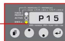
Abb. 15: Bedienfeld / DMX-Signal
